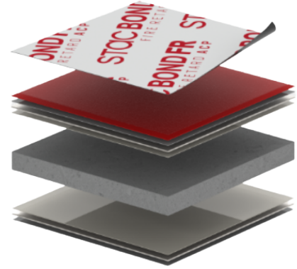
PANNEAU COMPOSITE ALUMINIUM IGNIFUGE
